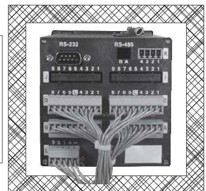
Schalttafel Ausschnitt: 91 x 90 mm
